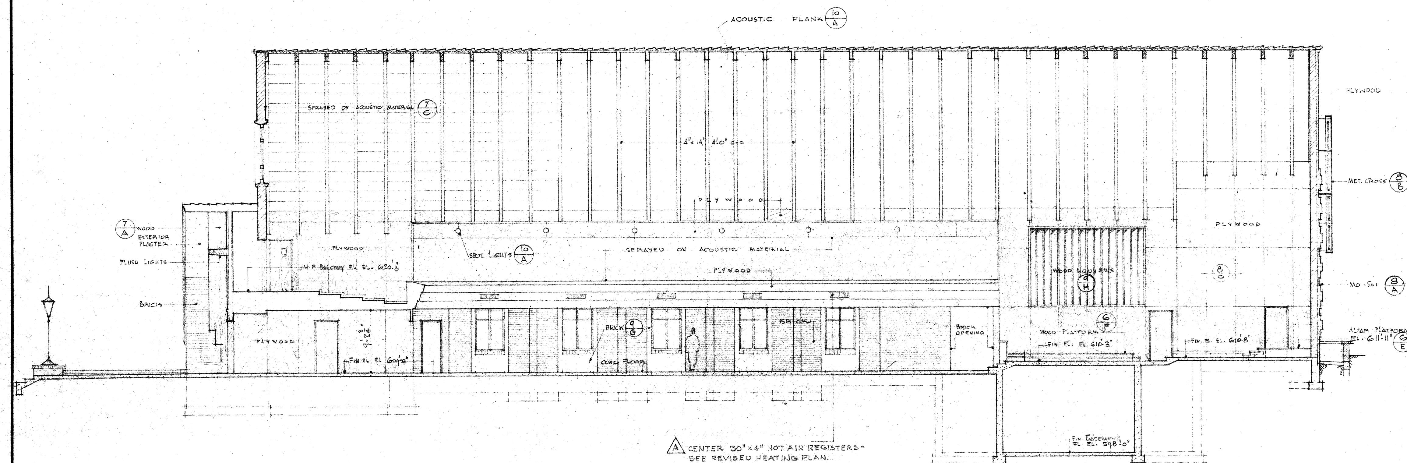
LONGITUDINAL SECTION A A
